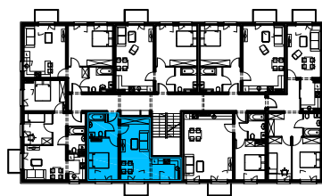
RZUT 1 PIĘTRA
