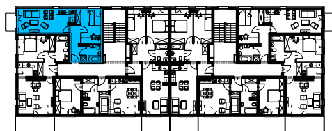
RZUT 2 PIĘTRA
