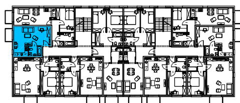
RZUT 1 PIĘTRA
