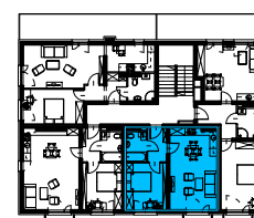
RZUT 2 PIĘTRA
