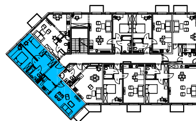
RZUT 1 PIĘTRA
