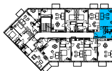
RZUT 1 PIĘTRA
