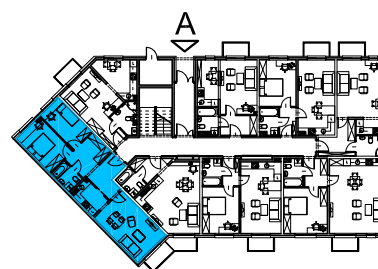
RZUT PARTERU
