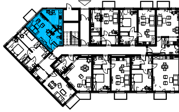
RZUT PARTERU
