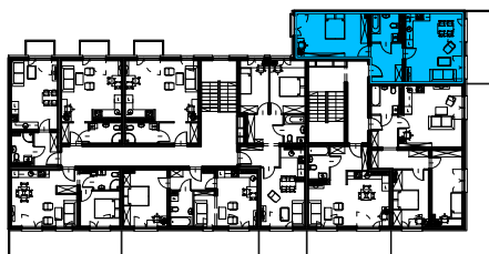
RZUT 2 PIĘTRA
