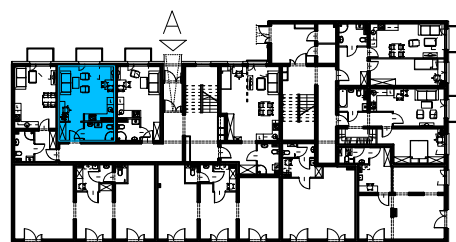
RZUT PARTERU
