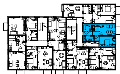
RZUT 1 PIĘTRA
