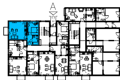
RZUT PARTERU
