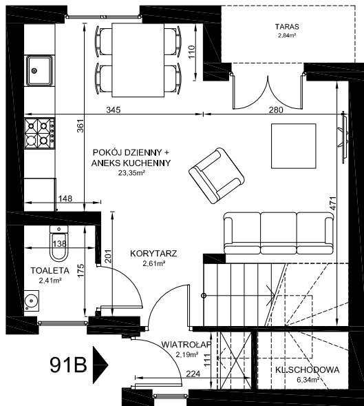
RZUT PARTERU
