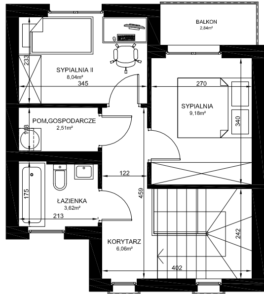
RZUT PIĘTRA
