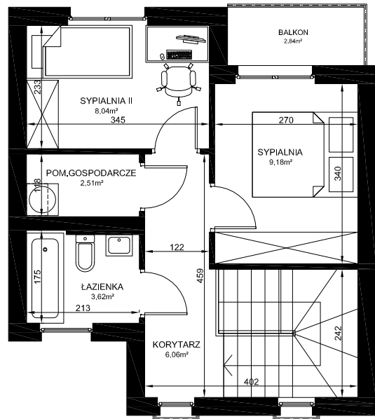
RZUT PIĘTRA
