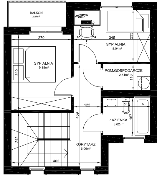
RZUT PIĘTRA
