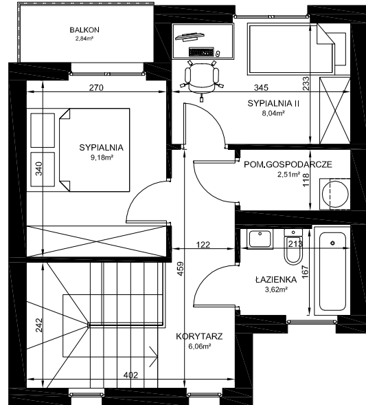
RZUT PIĘTRA
